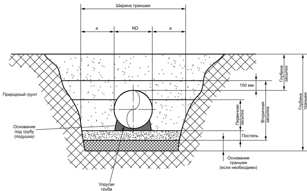
Рисунок 1. Схема укладки трубопровода.
